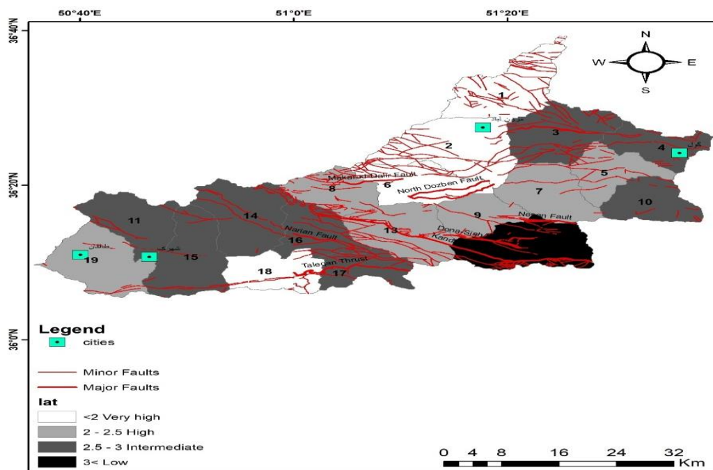
شکل ۵. نقشه پهنه‌بندی گستره مورد مطالعه براساس سطح شاخص زمین‌ساخت فعال نسبی (lat)
