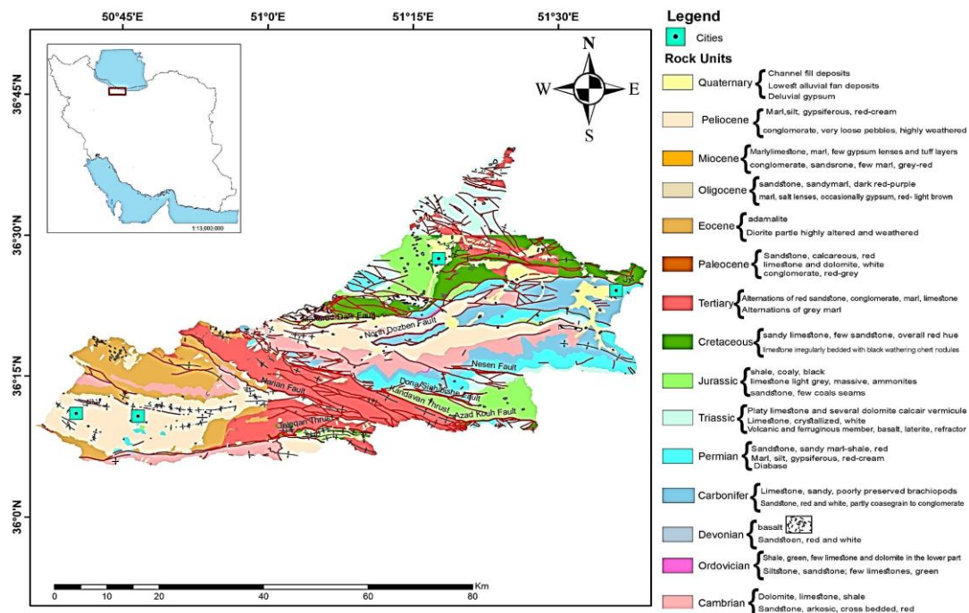
شکل ۱. نقشه زمین‌شناسی منطقه مورد مطالعه
