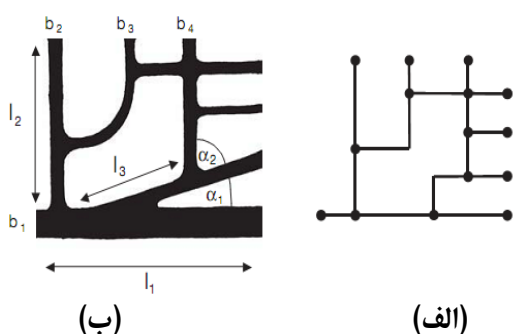
شکل ۲. (الف) پیکربندی و (ب) ترکیب شبکه
