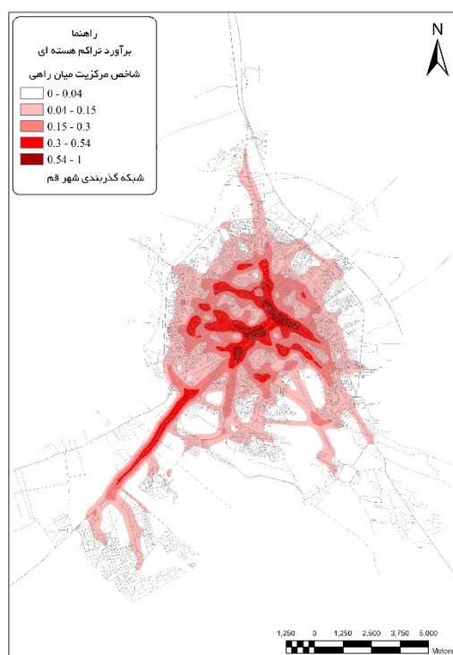
شکل ۷. تراکم مرکزیت میان‌راهی شبکه گذر بندی شهر قم مأخذ: یافته‌های تحقیق
